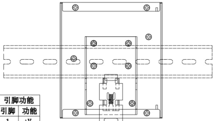
左视图
